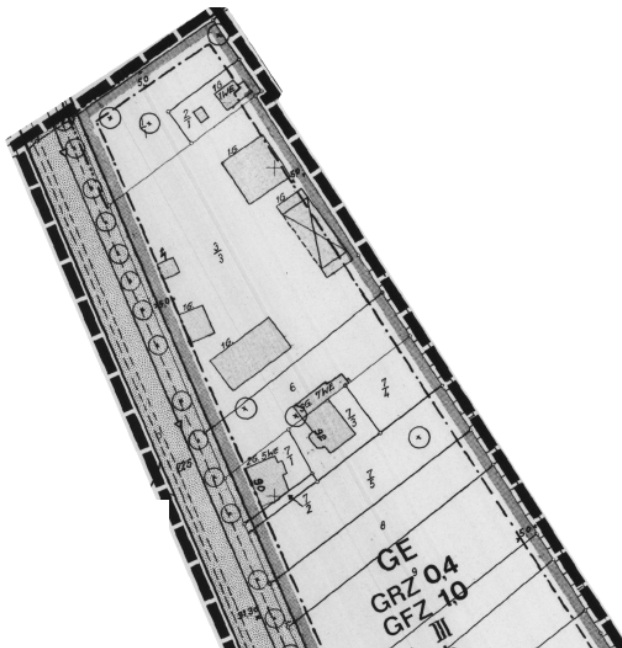
Ausschnitt aus dem Bebauungsplan
